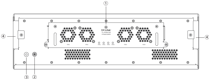
图1-4 TL-NR9700-B02后面板示意图
